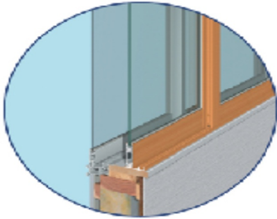
メルツエンサッシの納まり図 (窓枠に取り付けます)
