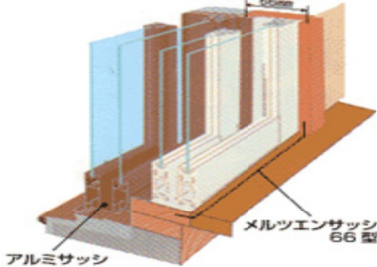
メルツエンサッシの納まり図 (窓枠に取り付けます)
